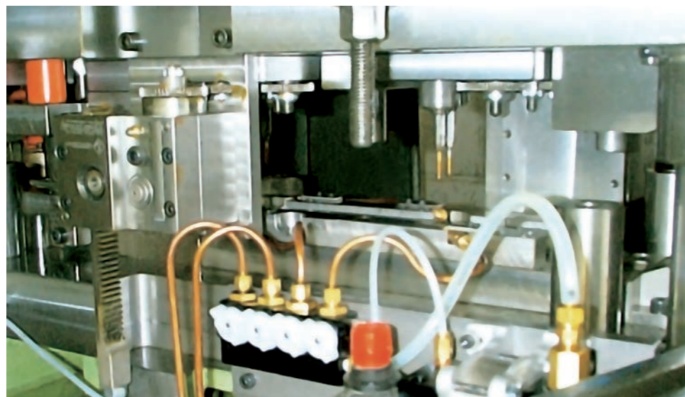
Maschiatrice ribaltata di 180°. Soluzione suggerita per stampi con corse lunghe (oltre 300-350 mm) Tapping unit at 180° overturned. This solution is suggested by dies with long runs (more than 300-350 mm) Gewindeformeinheit um 180 Grad. Lösungsvorschlag für Werkzeuge mit langen Hub (More Than 300-350 mm)
